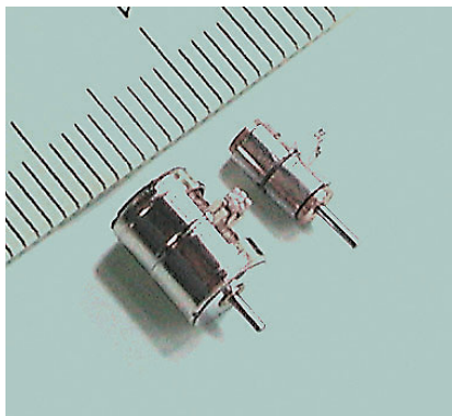
直径3mmステッピングモーター（写真右）と 直径6mmステッピングモーター
